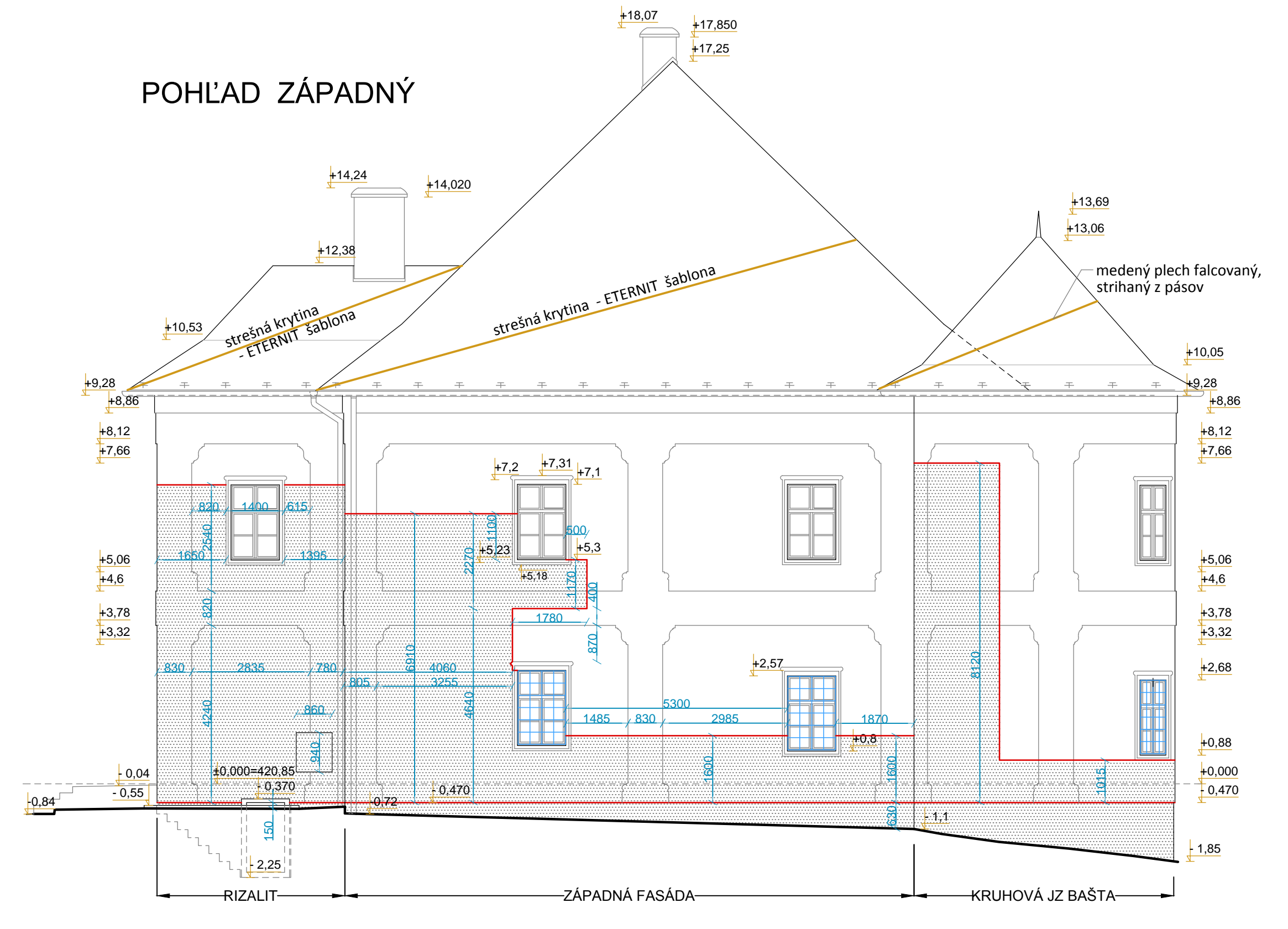
PRÍLOHA č.6 KAŠTIEĽ KRIVANY, M=1:100 POHĽAD JUŽNÝ A ZÁPADNÝ -ROZSAH SANAČNEJ OMIETKY
