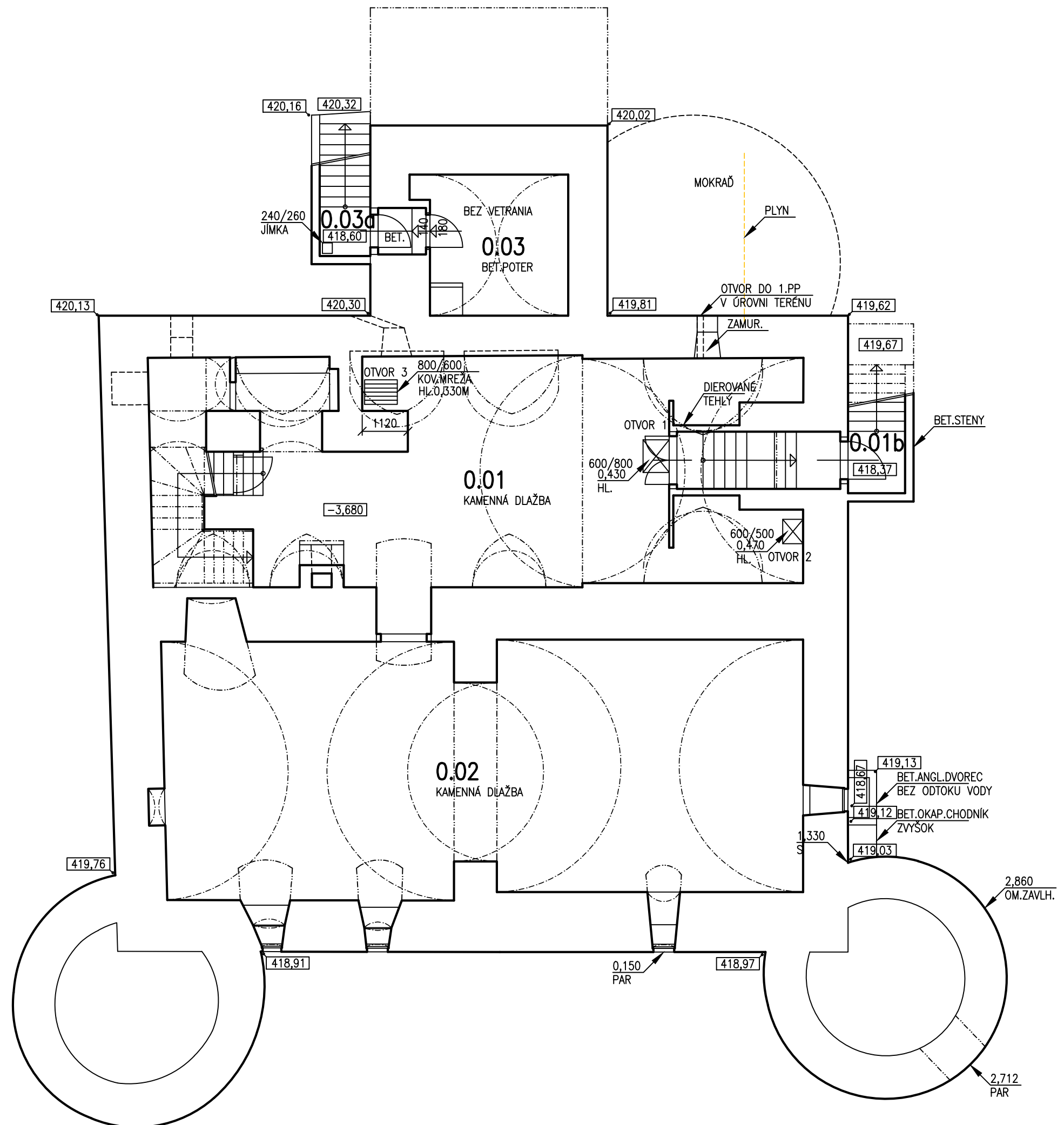
PRÍLOHA č.1 KAŠTIEĽ KRIVANY PÔDORYS 1.PP- PRIESKUM, M=1:100
